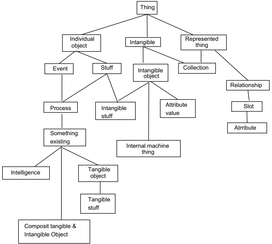
Fig. 6.3 World ontology
