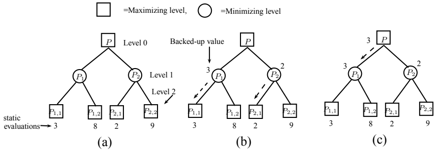
Fig. 11.8 MINIMAX search
